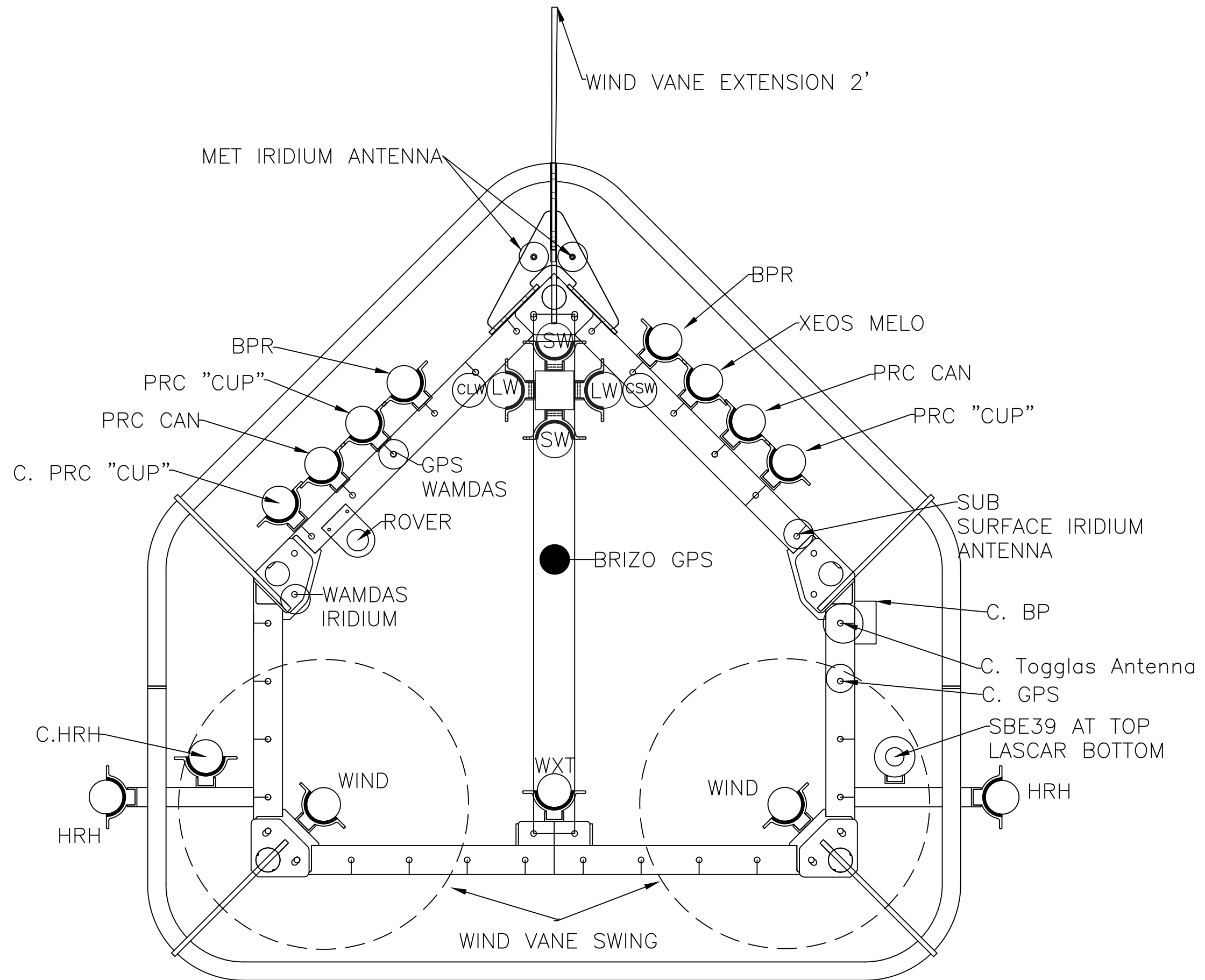
NTAS 18 TOWER TOP V3
